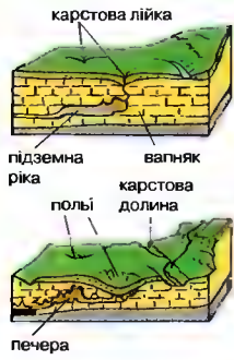
Карст Розвиток карстових форм
